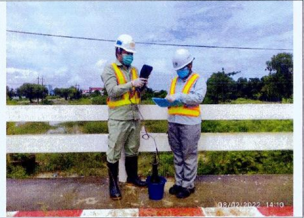
မြေပေါ်ရေ နမူနာယူသည့်နေရာ-၂ (SW-2) ၌ ရေနမူနာရယူခြင်းနှင့်တိုင်းတာခြင်း
