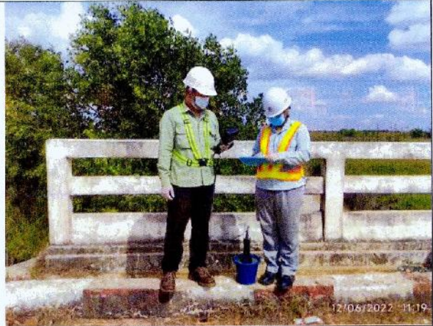
မြေပေါ်ရေ နမူနာယူသည့်နေရာ-၄ (SW-4) ၌ ရေနမူနာရယူခြင်းနှင့်တိုင်းတာခြင်း
